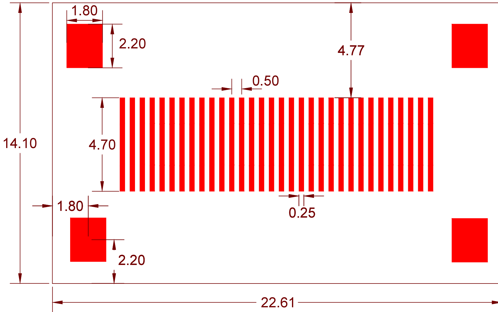
COPPER LAYER
